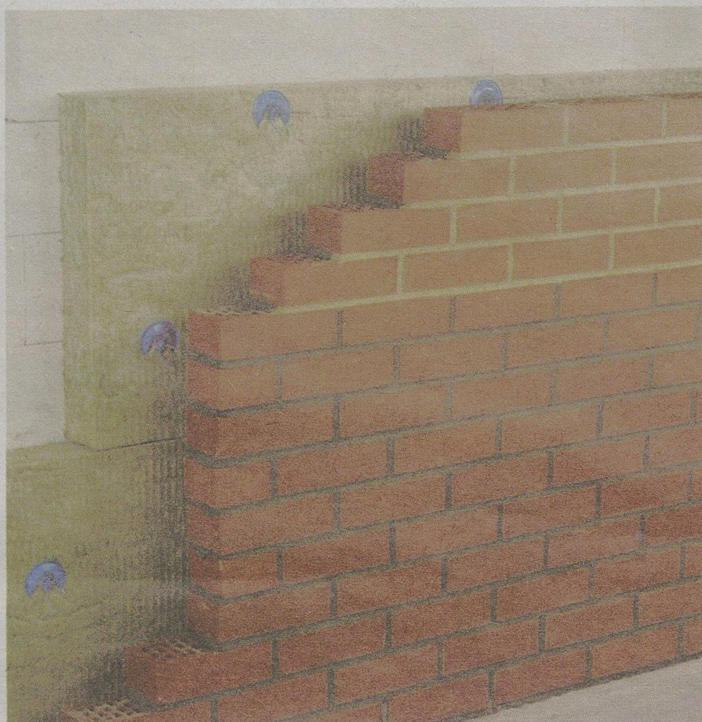
Fragment ściany ocieplonej metodą „lekko sucho”
