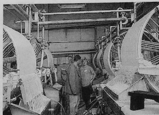
Zmodernizowana suszarnia skrobi w krochmalni Pepeesu
