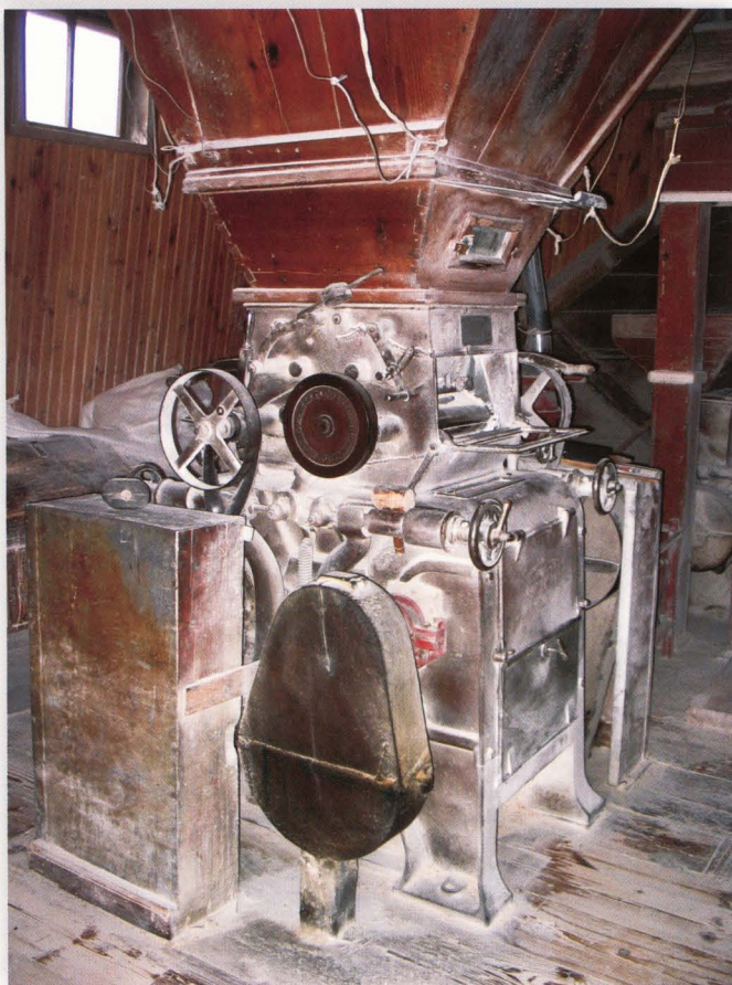
Stare Dolistowo. Wnętrze wiatraka z urządzeniami młyńskimi.
