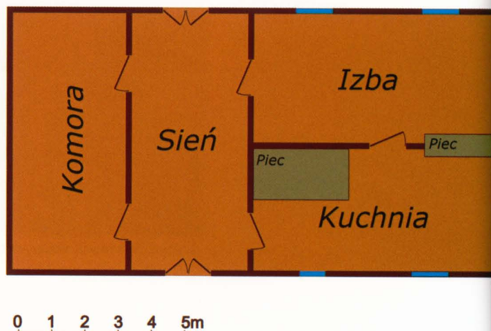
Lipszczany 12. Rozplanowanie wnętrza domu.
