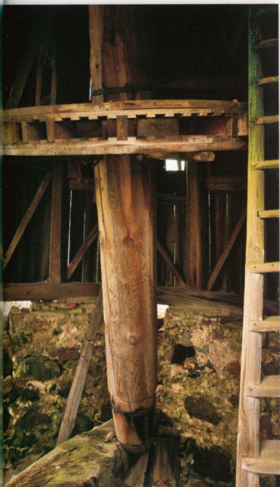
Stara Kamienna. Wnętrze wiatraka – koło trybowe na wale pionowym, zazębiające się z kołem cewkowym umieszczonym na wrzecionie złożenia kamieni młyńskich.
