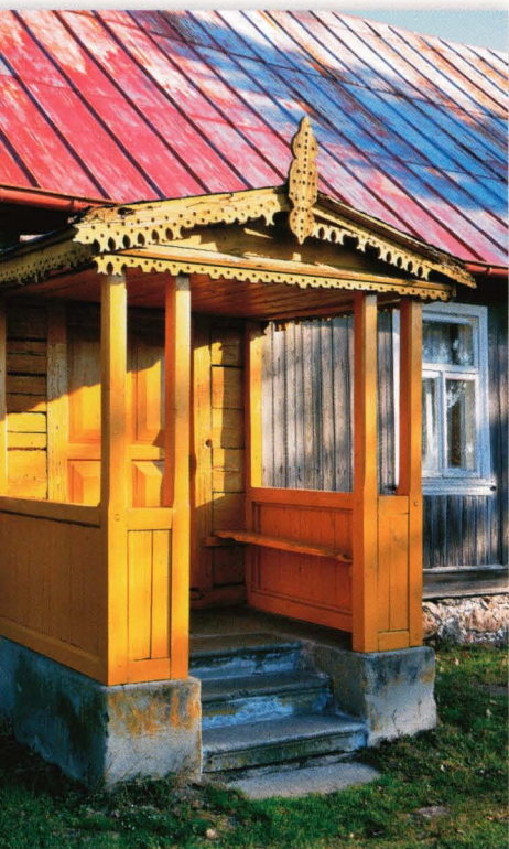
Goniądz, ul. Kościuszki 54. Daszek ganka z listwą podokapową i wiatrownicami od frontu. W miejscu łączenia się wiatrownic pazdur z profilowane wycięta krawędzią, zdobiony nieprzełotowymi otworami.
