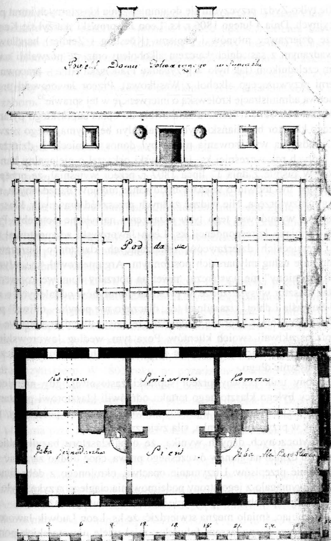
Ilustracja IX. Plan „domu folwarcznego” wykonany prawdopodobnie w 1806 r. przez opata Leona Jaworowskiego; APwB. Kamera Wojny i Domen, sygn. 1074, k. 81.
